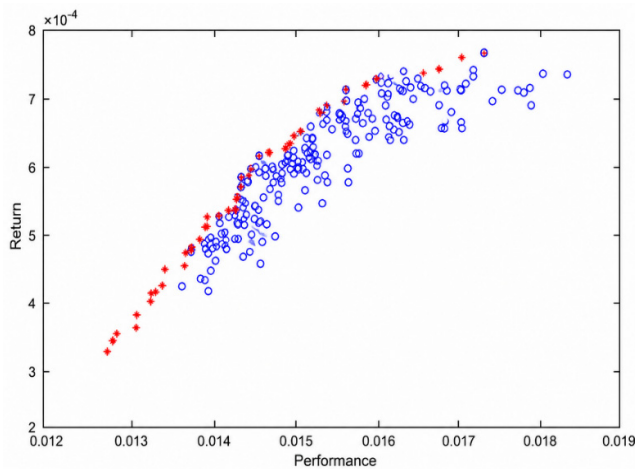
شکل ۲۰: بهینه‌سازی گیت‌های منطقی AND بر پایه موجبر پلاسمونی با برازش LSTM (قرمز رنگ) و بدون LSTM (آبی رنگ)
